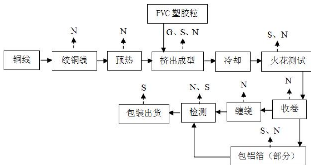
图 3-3 电线加工生产工艺及产污环节流程图
