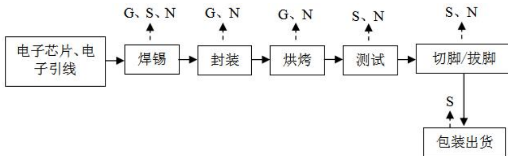
图 3-3 电子产品生产工艺及产污环节流程图
