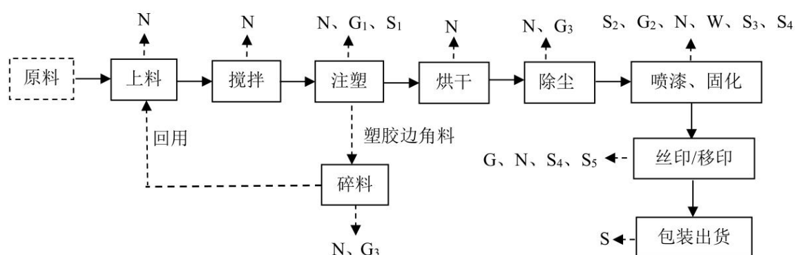
图 3-2 塑胶产品生产工艺及产污环节图
