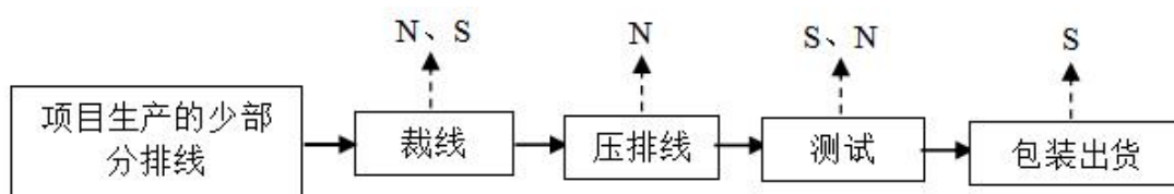
图 3-3 插头工艺及产污环节图
