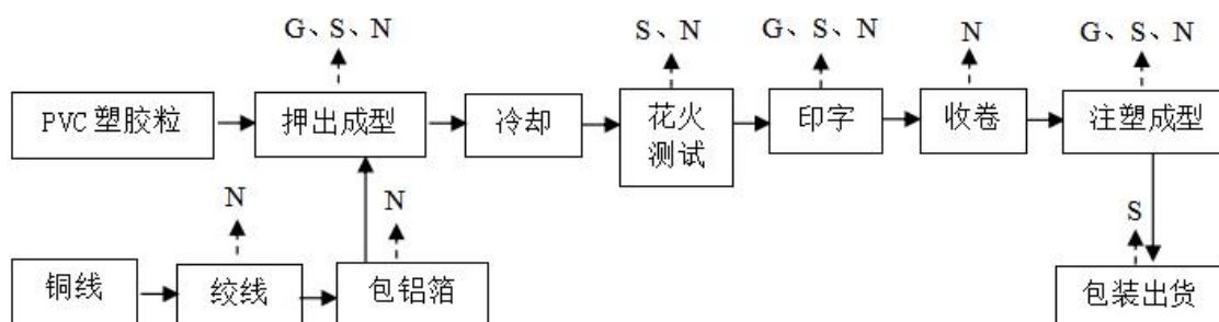
图 3-2 项目排线生产工艺及产污环节图
