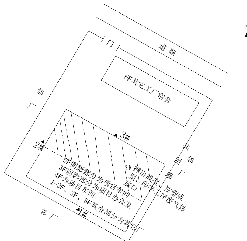
图 3-1 厂区平面布置及监测点位
