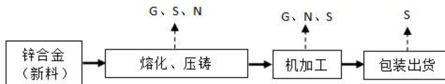
图 3-3 项目五金配件生产工艺及产污环节流程图
