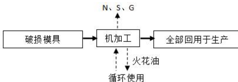
图 3-4 项目破损模具维修工艺及产污环节流程图
