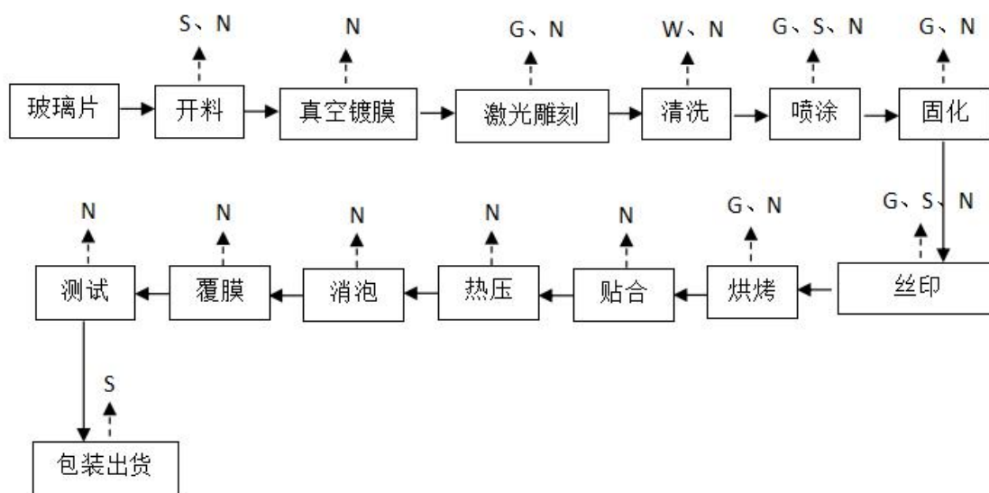
图 3-2 触摸屏生产工艺及产污环节图
